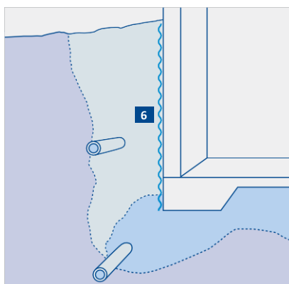
Fuktspärre med HD-polyeten
